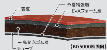
【BG5000断面図】
